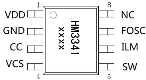
ESOP8
